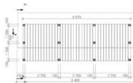
ПЛАН М 1:100
