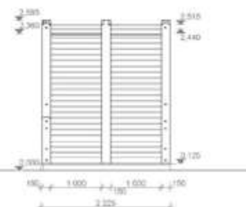
РАЗРЕЗ 2-2 М 1:50
